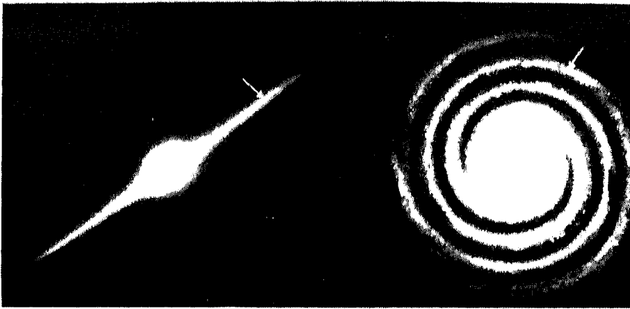
شكل ( 7 ) منظر جانبي لنظام درب التبانة . ويشير السهم الى موقع الشمس . لاحظ الشكل اللولبي الحلزوني للمجرة (2) .
